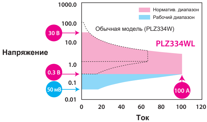
▲ Концептуальный чертеж рабочего диапазона
