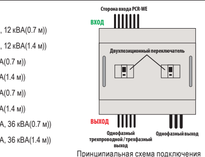
Принципиальная схема подключения
