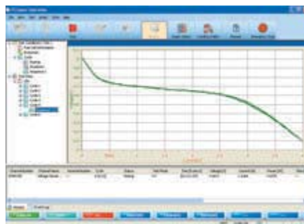
▲ Вольт-амперные характеристики
