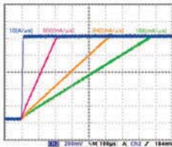
▲ Сдвиг формы волны тока в зависимости от переменной скорости нарастания
