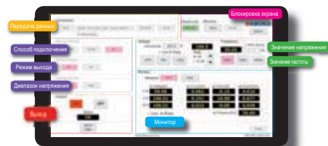
Экранный дисплей (главный экран)
