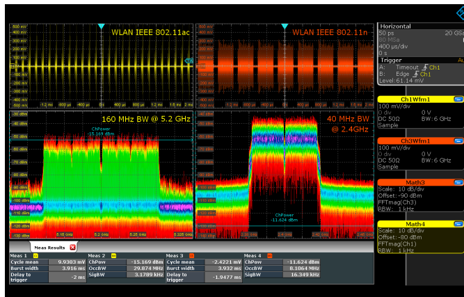
Многоканальный частотный анализ сигналов WLAN IEEE 802.11n и 11ac MIMO в осциллографе R&S®RTP
