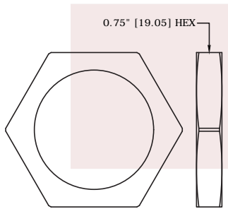
NUT
