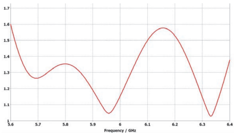
Порт V
