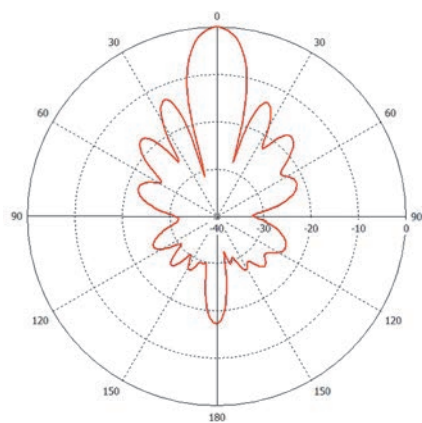
Горизонтальная плоскость
