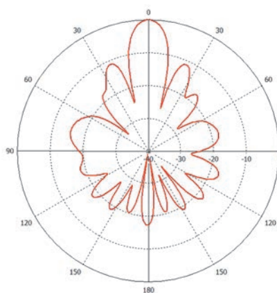
Вертикальная плоскость
