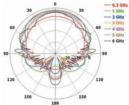
Горизонтальная плоскость
