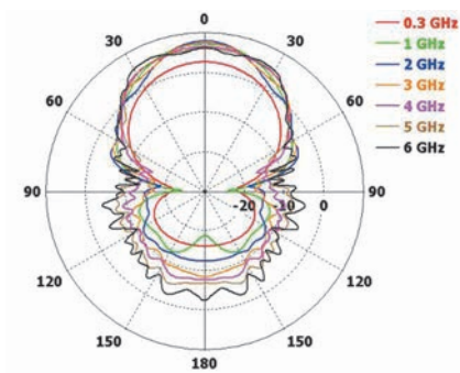
Вертикальная плоскость
