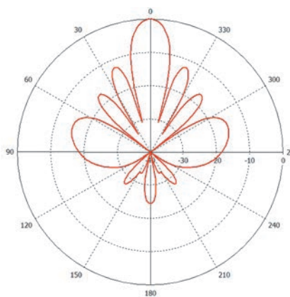
Вертикальная плоскость
