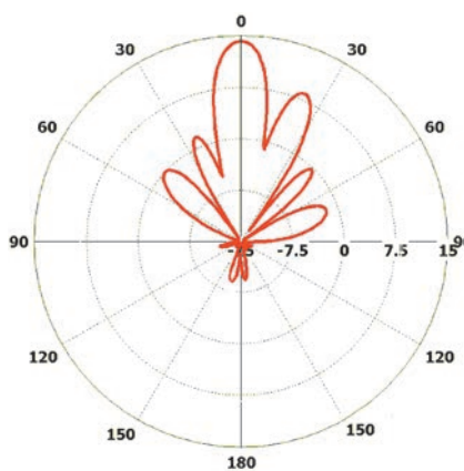
Вертикальная плоскость
