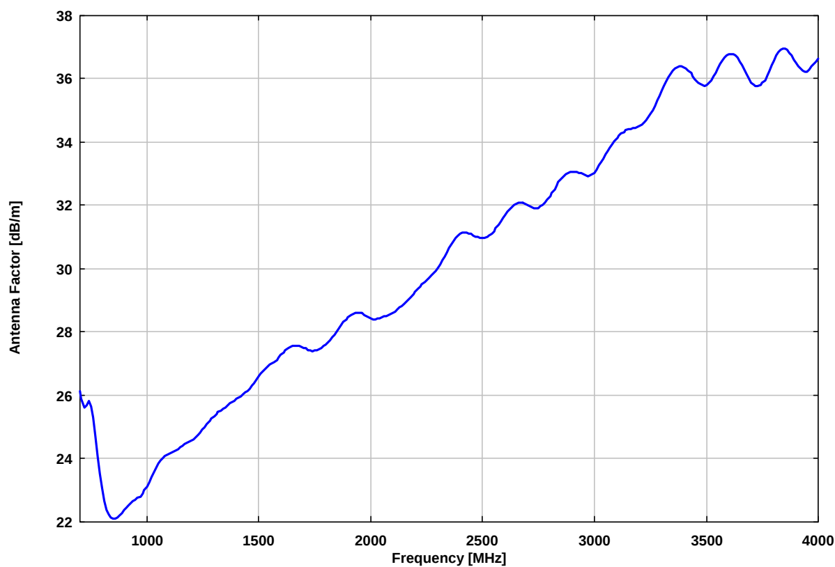
Antennenfaktor (k-Faktor):
