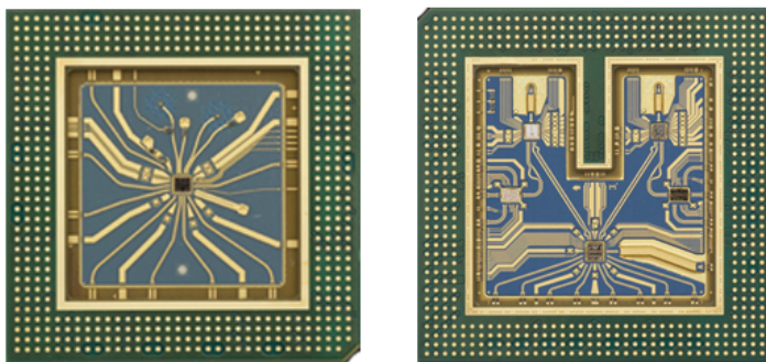
Специализированные многокристальные модули с индий-фосфидными кристаллами и запатентованная компанией Keysight технология корпусирования обеспечивают широкую полосу пропускания и малый уровень шумов.
